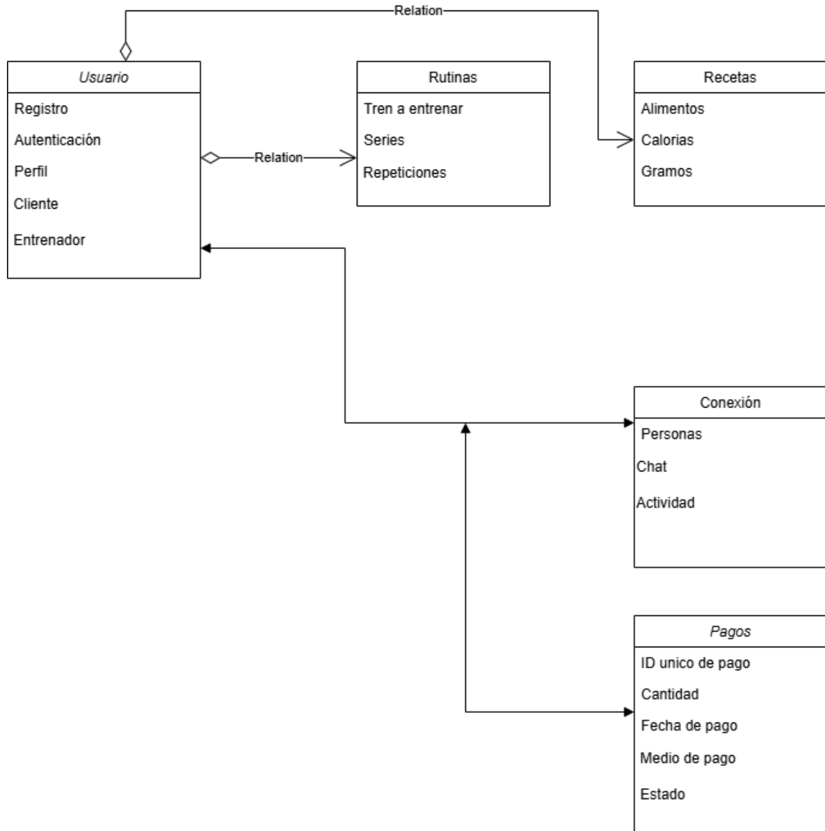
Diagrama 3 Paquetes
